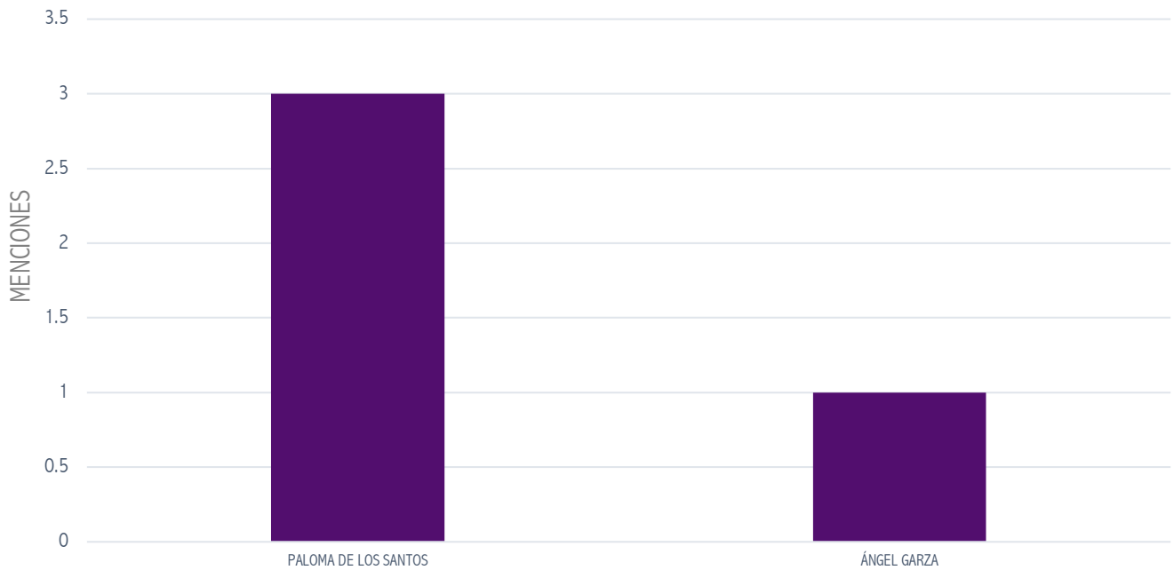
Figura 21: Monitoreo Cuantitativo en prensa escrita. Fuente: Análisis y Control de Medios SIMMCA 2023
